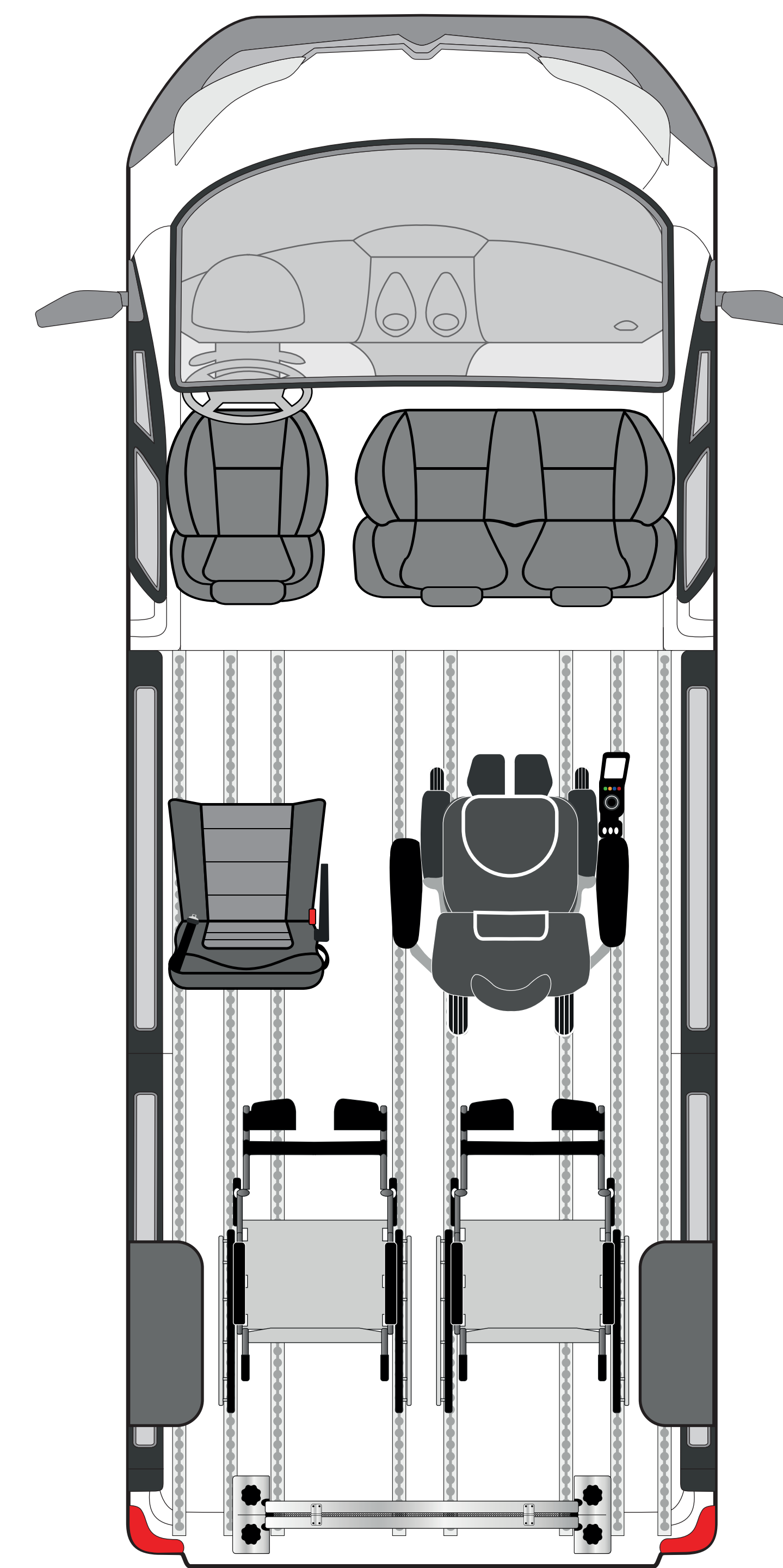
4 places + 3 Fauteuil roulant
