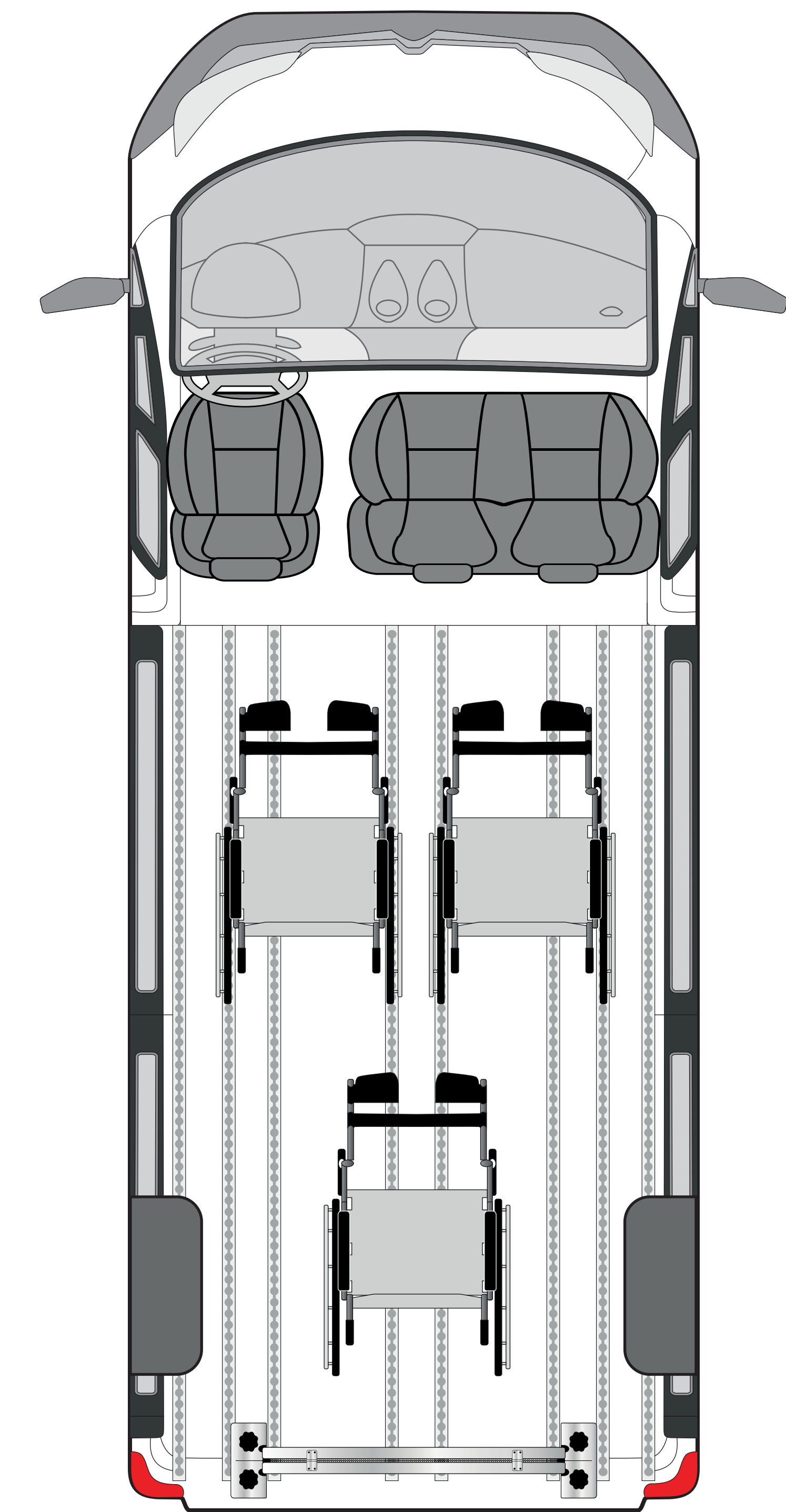
3 places + 3 Fauteuils roulants
